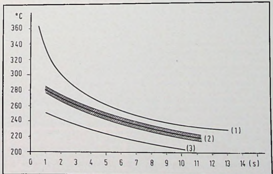
Bild 1. Löttemperatur in Abhängigkeit von der Lötzeit [4] 1 – LötKolbentemperatur für einen bestimmten LötKolbentyp 2 – Löttemperatur bei normaler Lötbarkeit mit Toleranzen 3 – Löttemperatur bei bester Lötbarkeit
