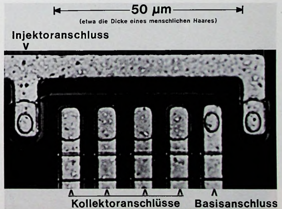
Bild 7. Mikrofotografie eines Multikollektor-Transistors mit vier Kollektorenanlässen, der das MTL-Grundbauelement ist
