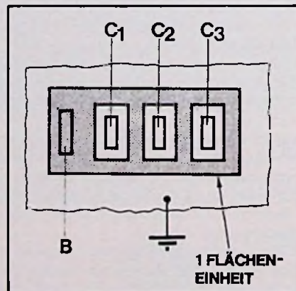
Bild 4. Beim inversen Multikollektor-Transistor fungieren die früheren Emittterzonen als Kollektor, und mehrere Regionen haben ein gemeinsames Basisgebiet
