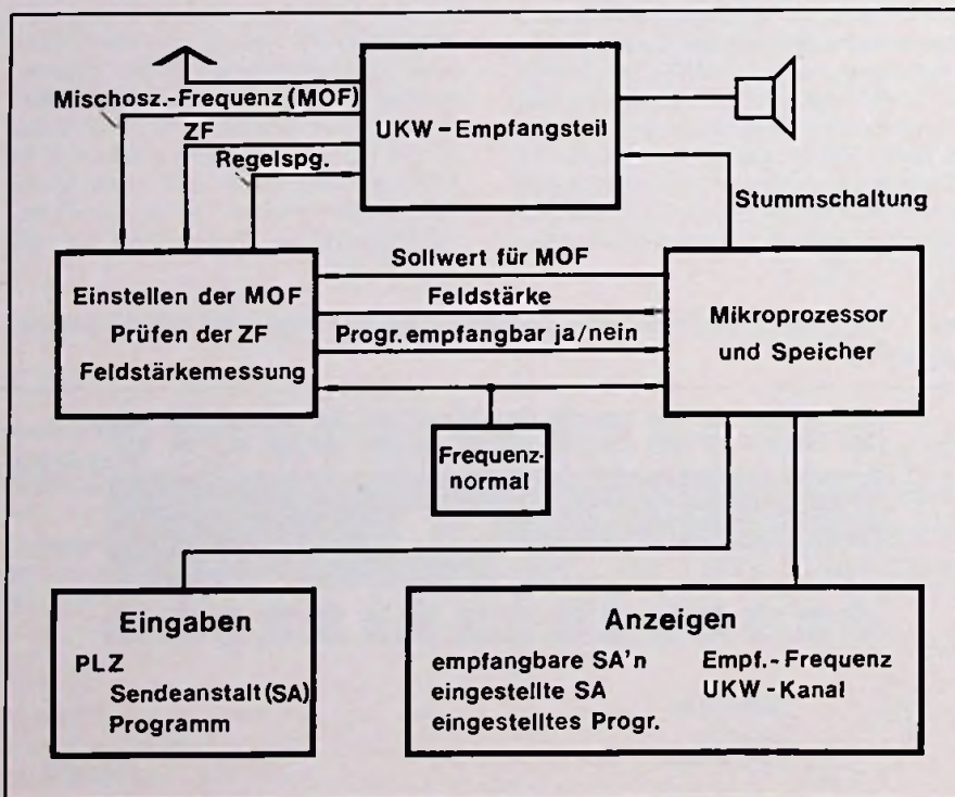
Bild 2. Funktionsplan des Entwicklungsmodells eines Empfängers mit Mikroprozessorsteuerung
