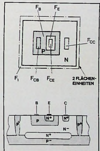
Bild 2. Draufsicht (oben) und Querschnitt (unten) eines NPN-Schalttransistors in konventioneller Bauart
