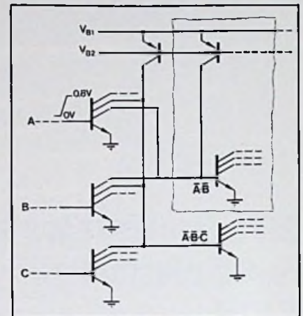
Bild 5. Logische Schaltung mit den noch getrennten PNP- und Multikollektor-NPN-Transistoren
