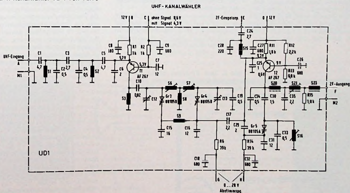
Bild 1. Kanalwähler VD 1 von Valvo
