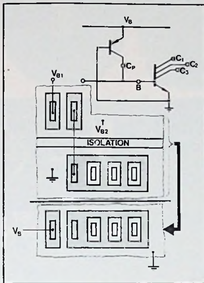
Bild 6. Schaltbild (oben) und Layout-Bild (unten) der Verschmelzung von PNP- und NPN-Transistoren zur Merged Transistor Logic (MTL)
