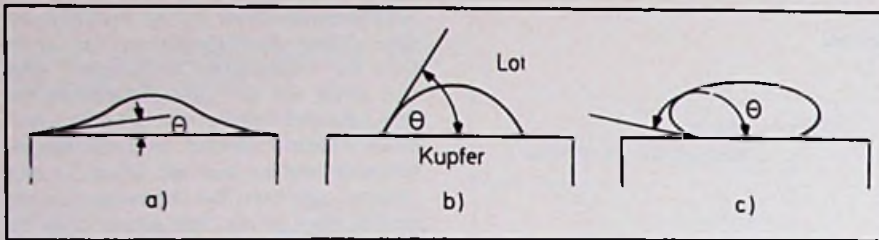
Bild 2. Benetzungswinkel \Theta und Grad der Benetzung a – vollständige Benetzung b – teilweise Benetzung ( \Theta größer als 70^\circ ) c – vollständige Nichtbenetzung ( \Theta ungefähr 180^\circ )
