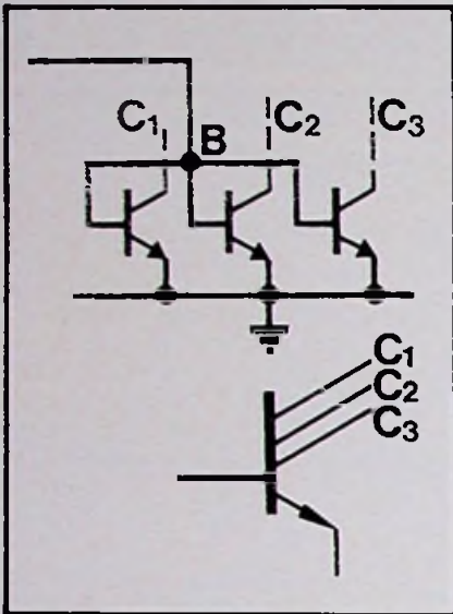
Bild 3. In einfachen Logikschaltungen haben kleinere Gruppen von 2 bis 4 Transistoren nicht nur gemeinsame Emittter, sondern auch eine gemeinsame Basis
