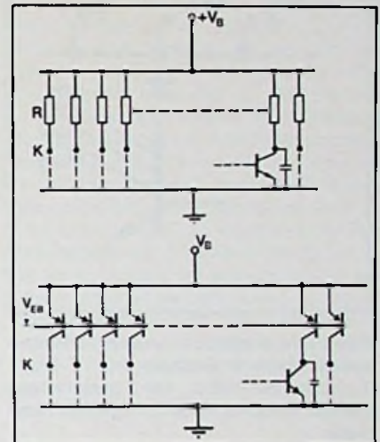
Bild 1. Prinzipschaltbild digitaler Schaltkreise mit ohmschem Widerstand (oben) und PNP-Transistor (unten) als Lastelement
